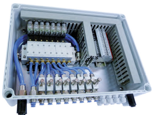
Riadiaci box s elektricky riadenými ventilmi pre prevádzku kŕmiacich zariadení
